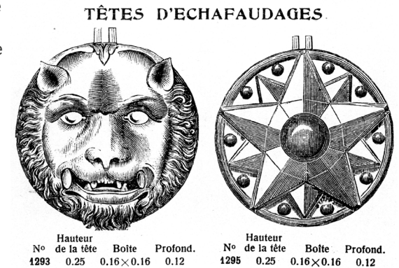
Modèle de couvercle de boudin en fonte Album des Articles de Bâtiments et de Jardins, Fonderie Nestor Martin ; succursales à Molenbeek-Saint-Jean (1911) ©Coll. AAM
