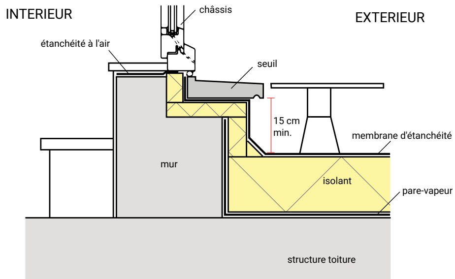
Relevé d'étanchéité d'une toiture aménagée en terrasse
