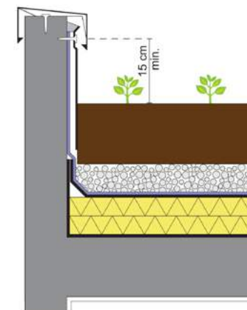
Relevé d'étanchéité le long de l'acrotère sur une toiture verte
