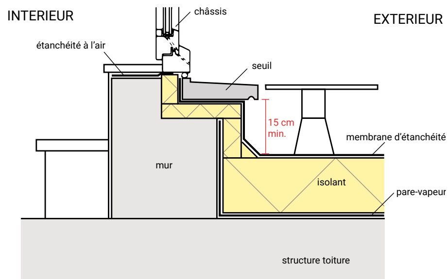
Relevé d'étanchéité sous un seuil de porte / porte-fenêtre
