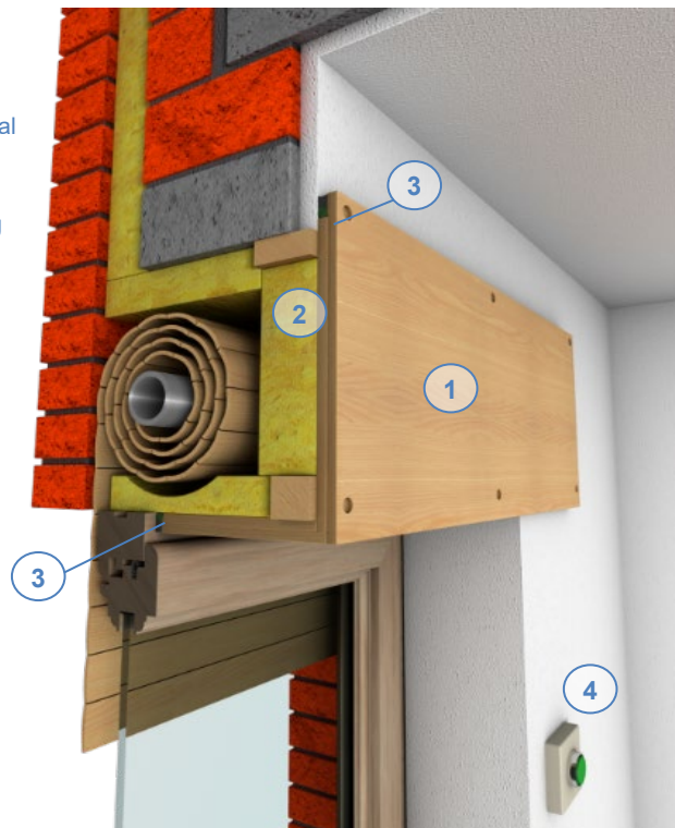
Figuur 32 : Geïsoleerde rolluikkast
