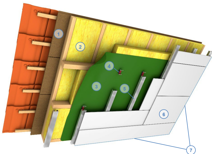
Figuur 60 : Zadeldak
