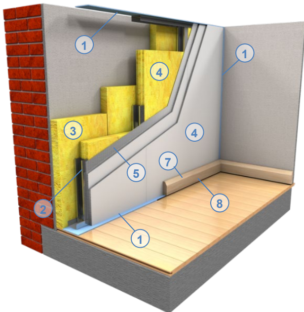
Figuur 32 : Bekleding op onafhankelijke draagstructuur gecombineerd met thermische isolatie
