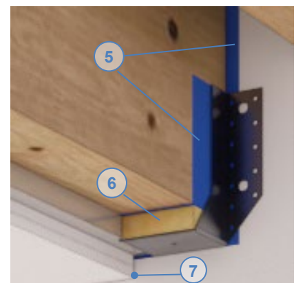
Figuur 19: schoen met een dempende laag en gevoerd met ontkoppelingsmateriaal
